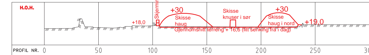
Snitt A
