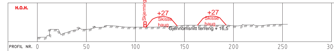
Snitt D
