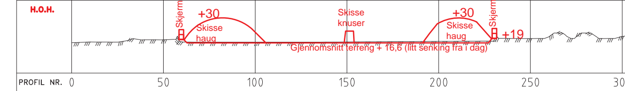
Snitt B
